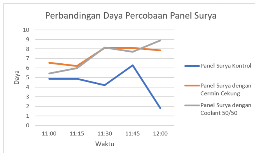
4.3 Grafik Perbandingan Daya Percobaan Panel Surya
