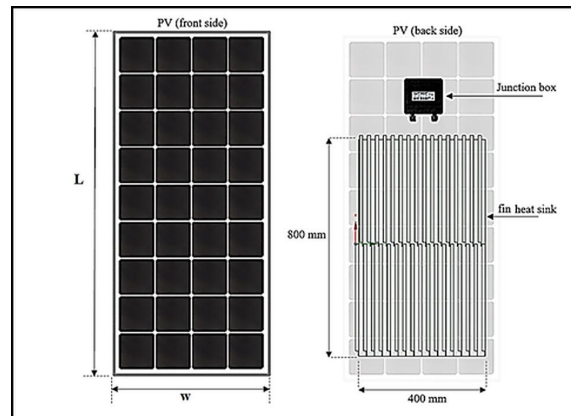
2.8 Sistem pendinginan panel surya menggunakan heatsink
