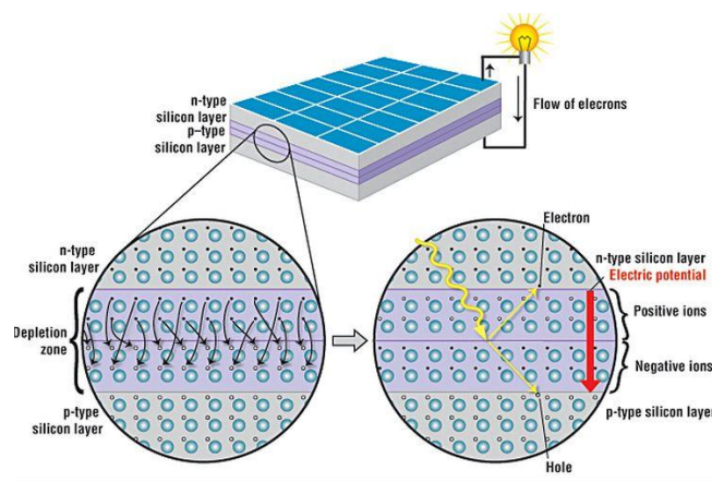
2.2 Prinsip kerja sel surya
