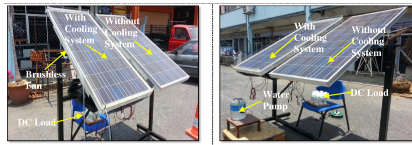
2.7 Sistem pendinginan panel surya menggunakan water cooling system dan kipas
